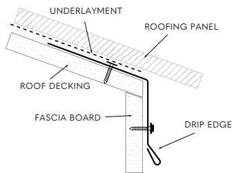
DRIP EDGE
